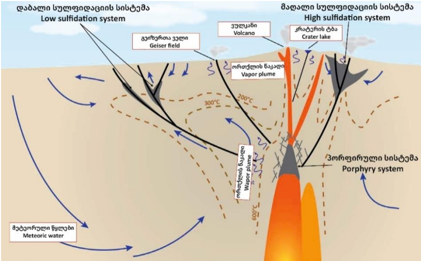
სურ. 1. კუნძულთა რკალების მადანწარმოქმნილი სისტემების მოდელი (Thomsen, 2015).
