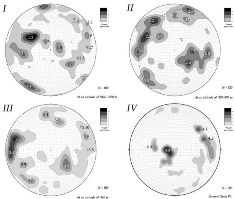
სურ.1. მუშევანის 2-ის (I, II, III) და კაზრეთის (IV) საბადოების მადნიანი ძარღვების პოლუსების სიმჭიდროვის იზოხაზები შმიდტის ტოლოფართი პროექციის ქვედა ნახევარსფეროზე.
